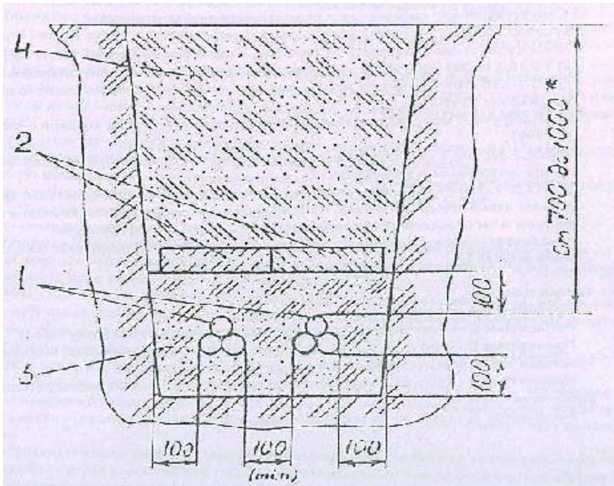
Рисунок 1 Прокладка кабелей 10 кВ в траншее, расстояние между кабельными линиями при параллельной прокладке в земле
